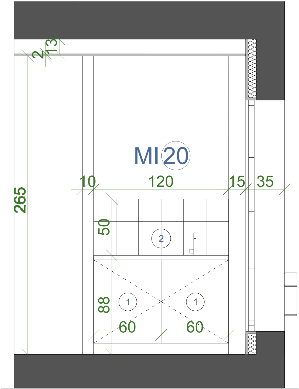
COUPE AA'
